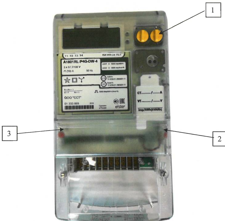
Рисунок 1 – Общий вид счетчика, схема пломбировки от несанкционированного доступа, обозначение места нанесения знака поверки
