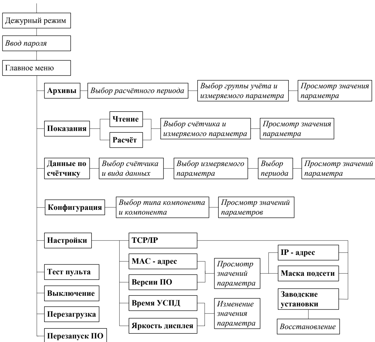
Схема №1. Структурная схема экранов меню дисплея пульта ввода/вывода.
