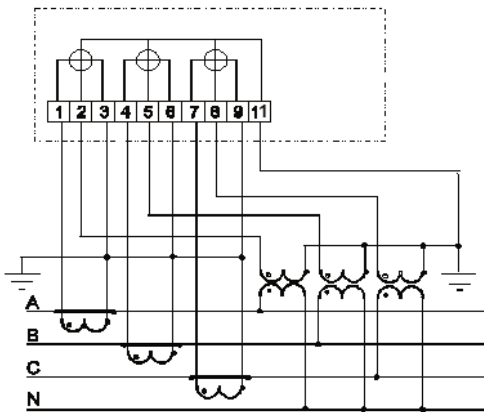
Рис.А.1 – Схема включения трехэлементного трансформаторного счетчика в четырехпроводную сеть с заземленной нейтралью.
