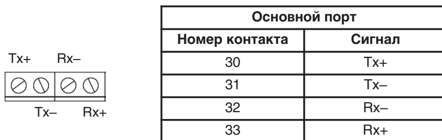
Рисунок 12.16 – Подключение интерфейса RS485 основной платы
