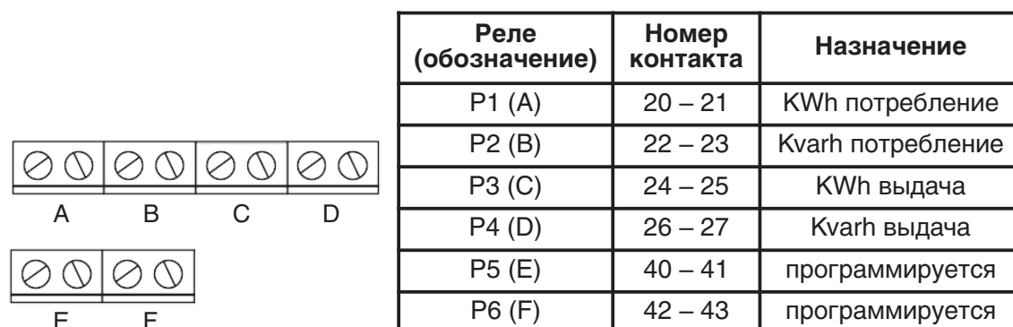
Рисунок 12.18 – Заводские установки импульсных каналов основной и дополнительной плат
