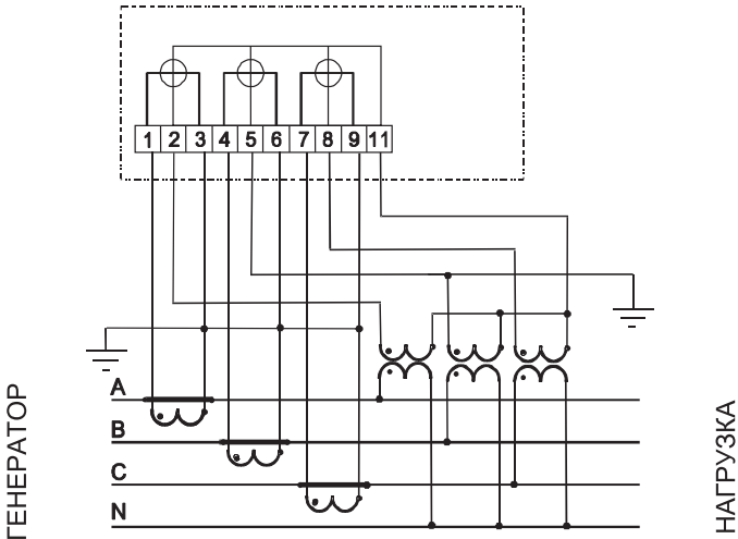
Рисунок 12.2 – Схема включения трехэлементного счетчика в четырехпроводную сеть с изолированной нейтралью заземленной фазой В
