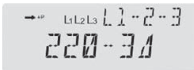
Рисунок 9.5 – Трехпроводная сеть с номинальным напряжением 220 В
