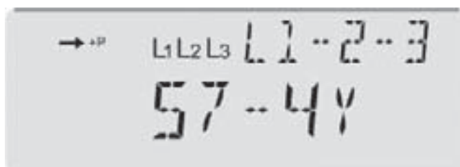
Рисунок 9.2 – Четырехпроводная сеть с номинальным напряжением 57,7 В
