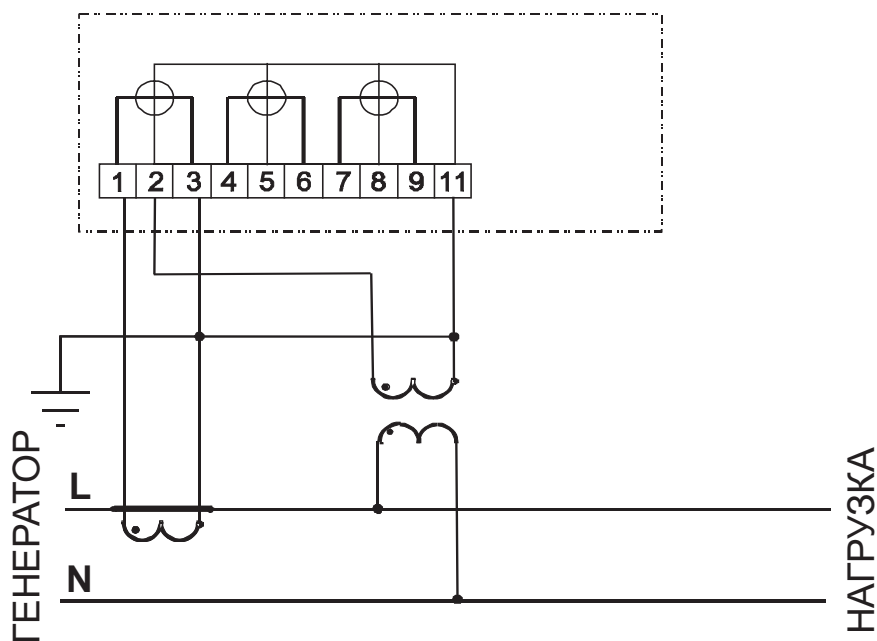
Рисунок 12.14 – Схема включения трехэлементного счетчика в однофазную сеть
