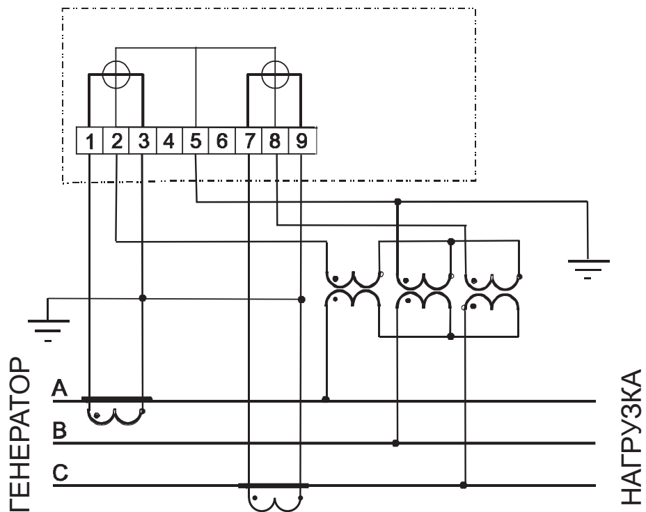
Рисунок 12.9 – Схема включения двухэлементного счетчика в трехпроводную сеть с тремя трансформаторами напряжения и заземленной фазой В
