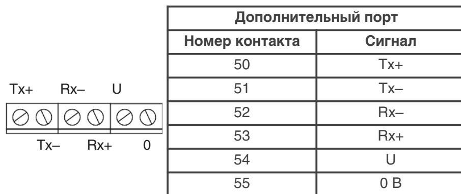
Рисунок 12.17 – Подключение интерфейса RS485 дополнительной платы
