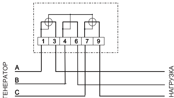
Рисунок 12.13 – Схема включения двухэлементного счетчика непосредственного включения в трехпроводную сеть напряжением 0,23 кВ
