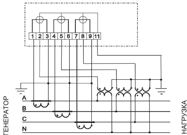
Рисунок 12.1 – Схема включения трехэлементного счетчика в четырехпроводную сеть с заземленной нейтралью
