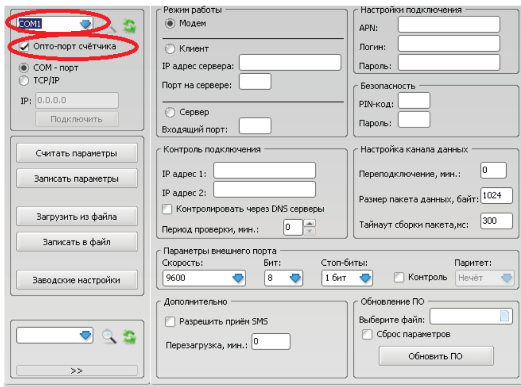
Рисунок 4 – Интерфейс конфигурационного ПО
